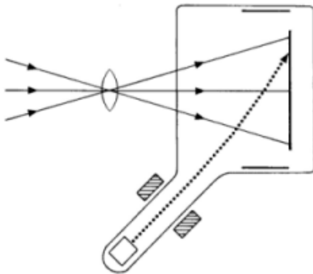
The iconoscope
