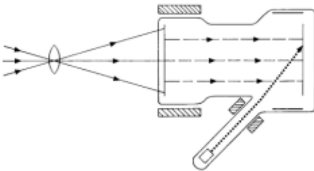
Super Iconoscope
