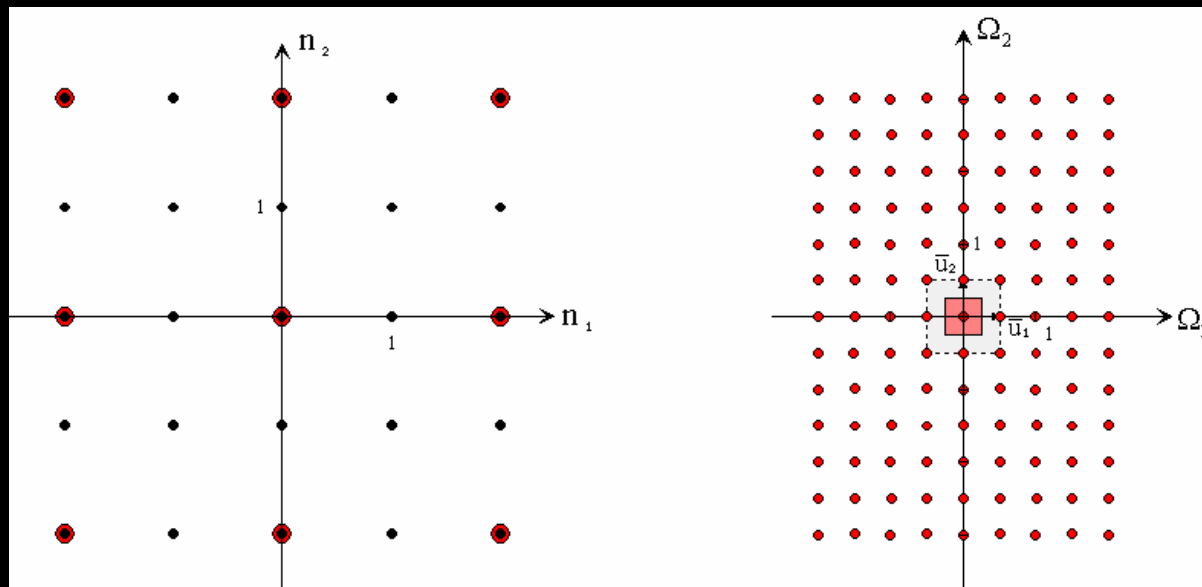
Submuestreo de las bandas R,B
