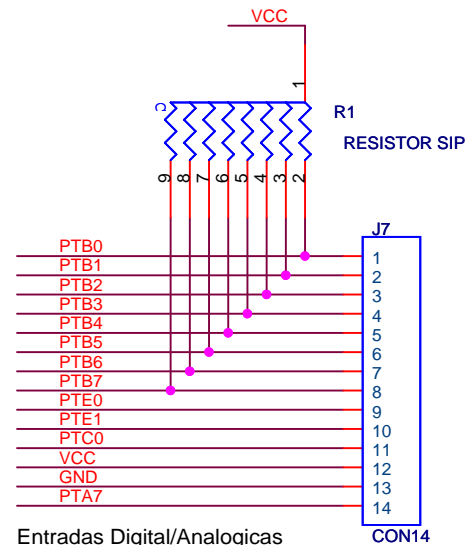
Entradas Digital/Analógicas (R de pull up internas al micro para entradas digitales. Para las entradas analógicas usar las que corresponda, conectandolas al zocalo del array de resistencias)
