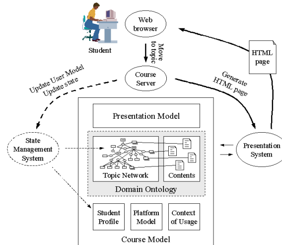
Fig. 2. Modelo del curso y arquitectura del sistema
