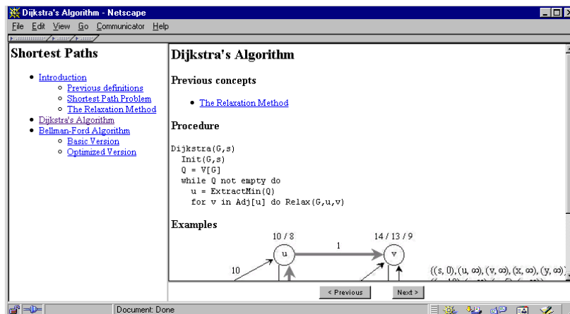
Fig. 1. Página web generada para un tópico de tipo Algoritmo
