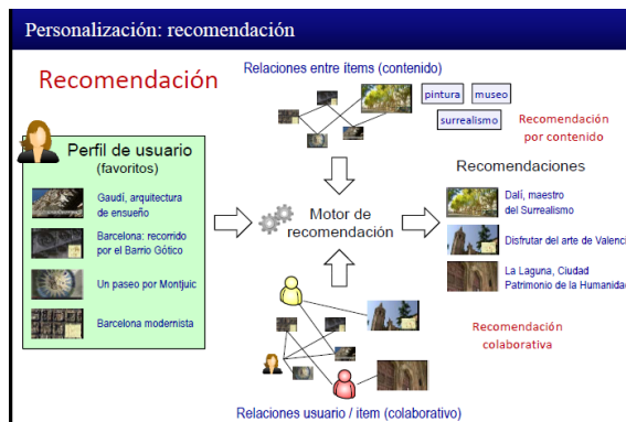
Figura 6: Recomendación
