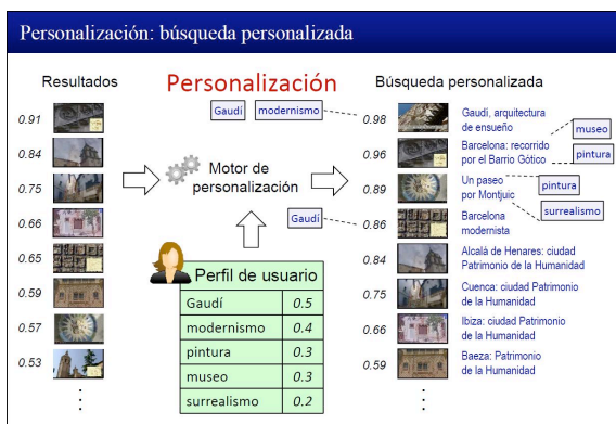
Figura 5: Personalización
